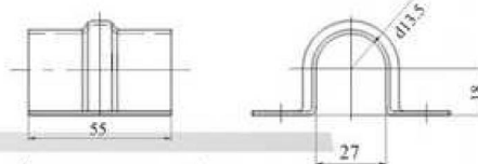
Опора трубы промежуточная верхняя d22 6305430-03
