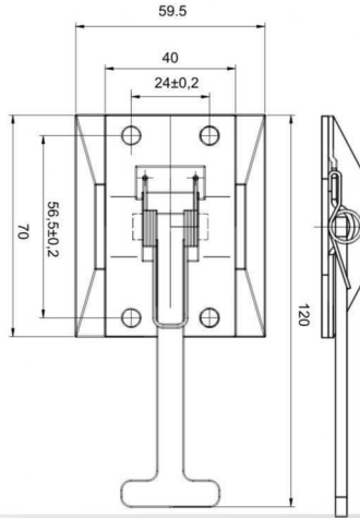
Фиксатор открытой двери ГРКП 456399.00
