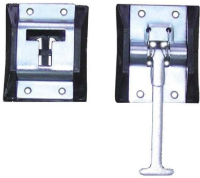
Фиксатор открытой двери ГРКП 456399.00
