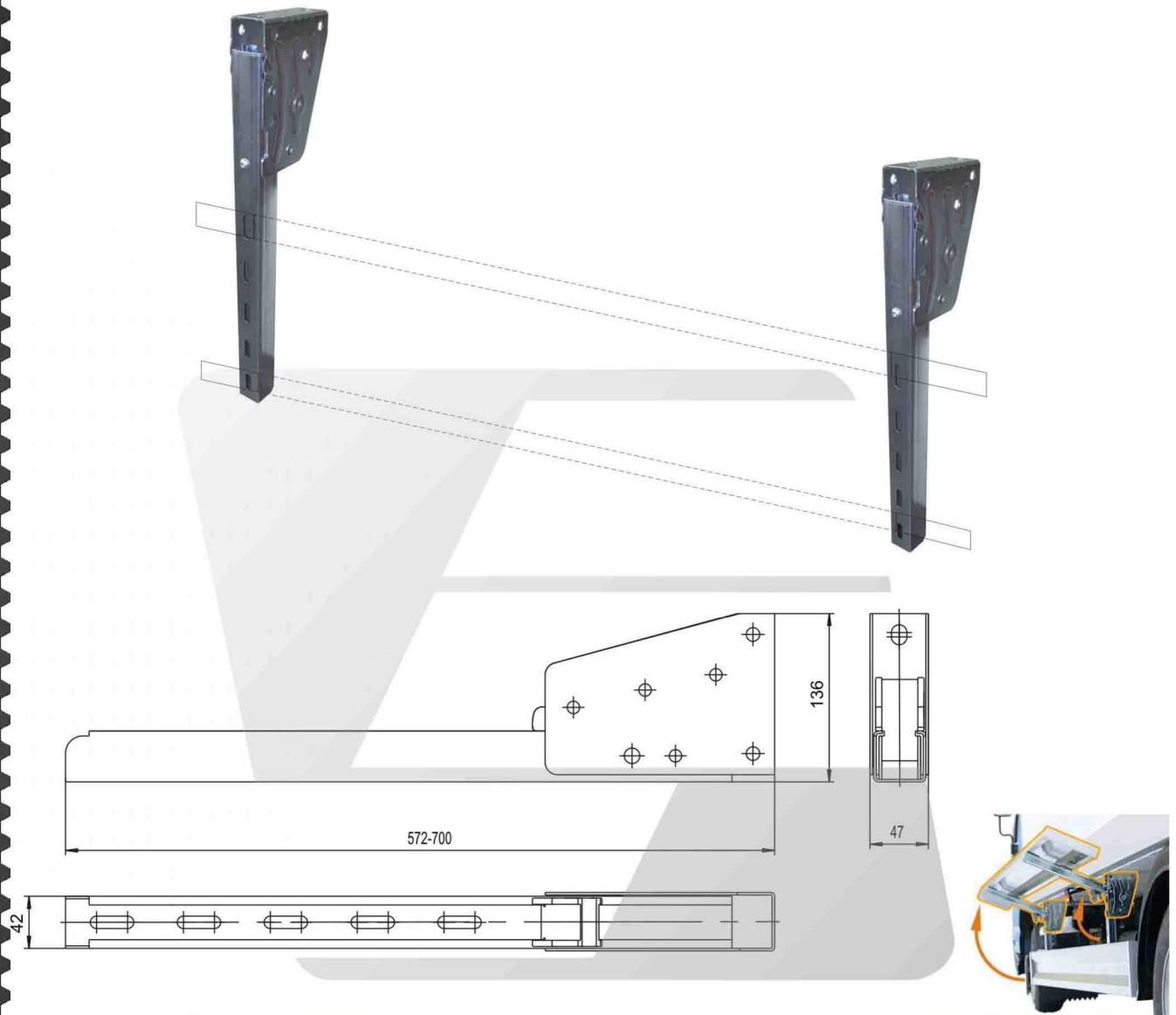
Кронштейн боковой защиты
